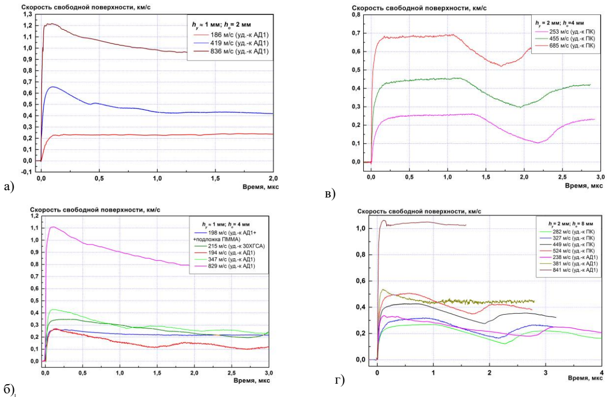
Рис. 1 – Профили скорости свободной поверхности образцов из поликарбоната марки ПК-ЭТ-3,5 с толщами ударник/образец: а) 1/2 мм, б) 1/4 мм, в) 2/4 мм, г) 2/8 мм
