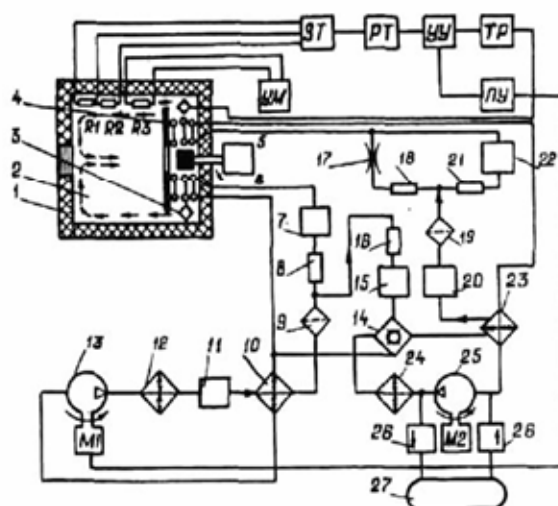
Рисунок 1.2 – Камера тепла и холода КТХ-0,4-65/155 1 – дверь; 2 – полезный объем; 3 – нагреватель; 4,6 – испарители; 5 – вентилятор; 7 – терморегулирующий вентиль; 8 – соленоидный клапан; 9,20 – фильтры; 10,14,26 – теплообменники; 11,23 – вентили; 12 – конденсатор теплотехнический; 13,22 – компрессоры; 15 – конденсатор-испаритель; 16,25 – термовентили; 17,19,21,24 – соленоидные вентили; 18 – дюза; 27 – емкость. ЗТ – задатчик температуры; РТ – регулятор температуры; УУ – устройство управления; ТР – тиристорный регулятор; ПУ – пусковое устройство; УМ – уравновешенный мост.
