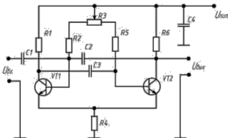
Рис. 116. Принципиальная электрическая схема генератора прямоугольных импульсов: C1 - К10-17-1нФ; C2 - C4 - К10-17-0,1нФ; C2 - 33 нФ-0,125; R1, R6 - 2 кОм; R2, R5 - 10 кОм; R4 - 200 Ом; C13 - 19а-0,125; R3 - 10 кОм; VT1, VT2 - КТ3102
